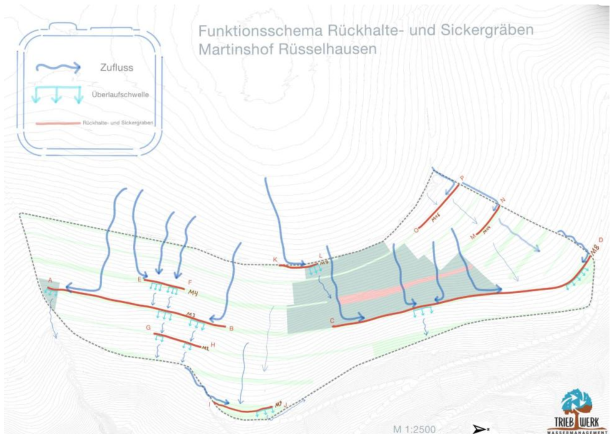
Abbildung 2: Funktionsschema inklusive Positionierung der Sedimentfanggräben
