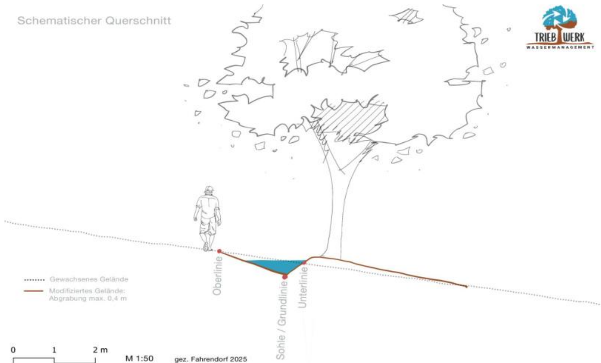
Abbildung 1: Aufbau der Sedimentfanggräben (schematische Darstellung)
